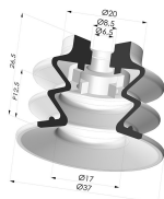
Ventosa 2.5 Fole Série 96 Ø 35MM
