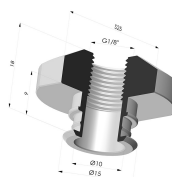
Inserto fêmea removível 1/8G
