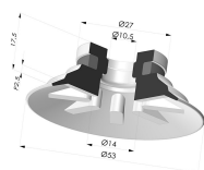
Ventosa plana Série 90 Ø 53 mm
