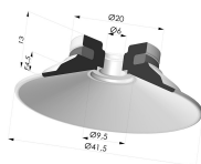
Ventosa plana Série 9 Ø 41,5 mm
