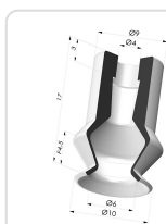
Ventosa 1.5 Fole Série 91 Ø 10,2 mm
