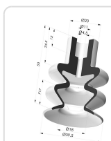
Ventosa 2.5 Fole Série 8B Ø 40MM
