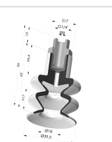
Ventosa 2.5 Fole Série 8B Ø 40MM
