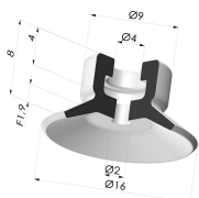
Ventosa plana da série PFG Ø 16 mm
