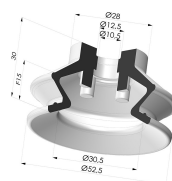
Ventosa 1.5 Fole Série 97B Ø 52,5 mm
