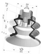
Ventosa 2.5 Fole Série 96C Ø 70MM
